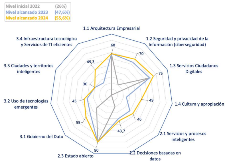
Gráfica 4. Evolución del modelo de capacidades de TI
