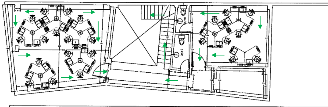
PLANTA PISO 2°
