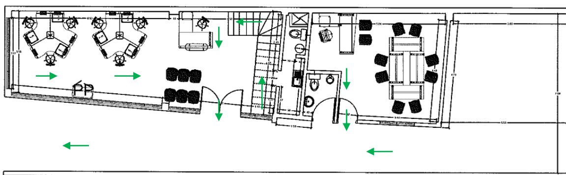
PLANTA PISO 1°
